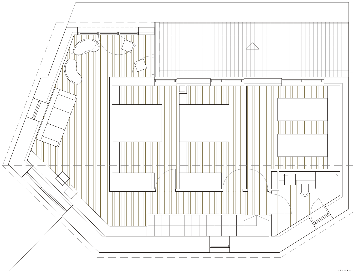
planta alta
