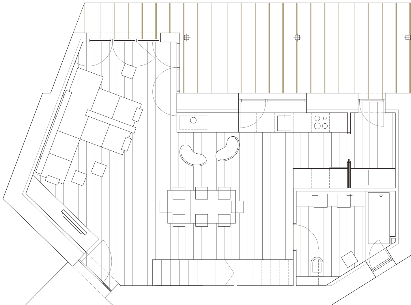
planta baja
