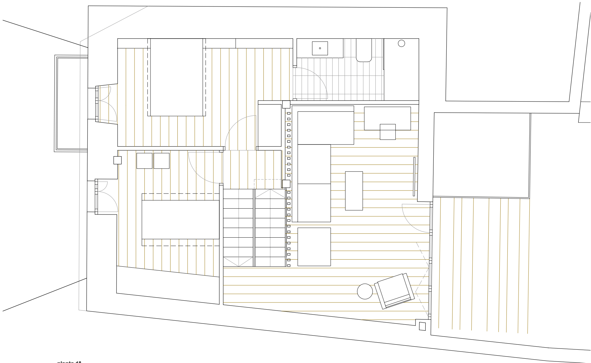
planta 1ª
