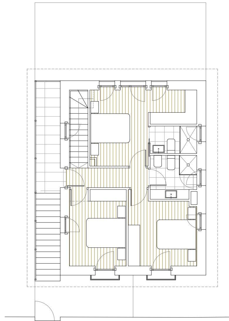
planta alta
