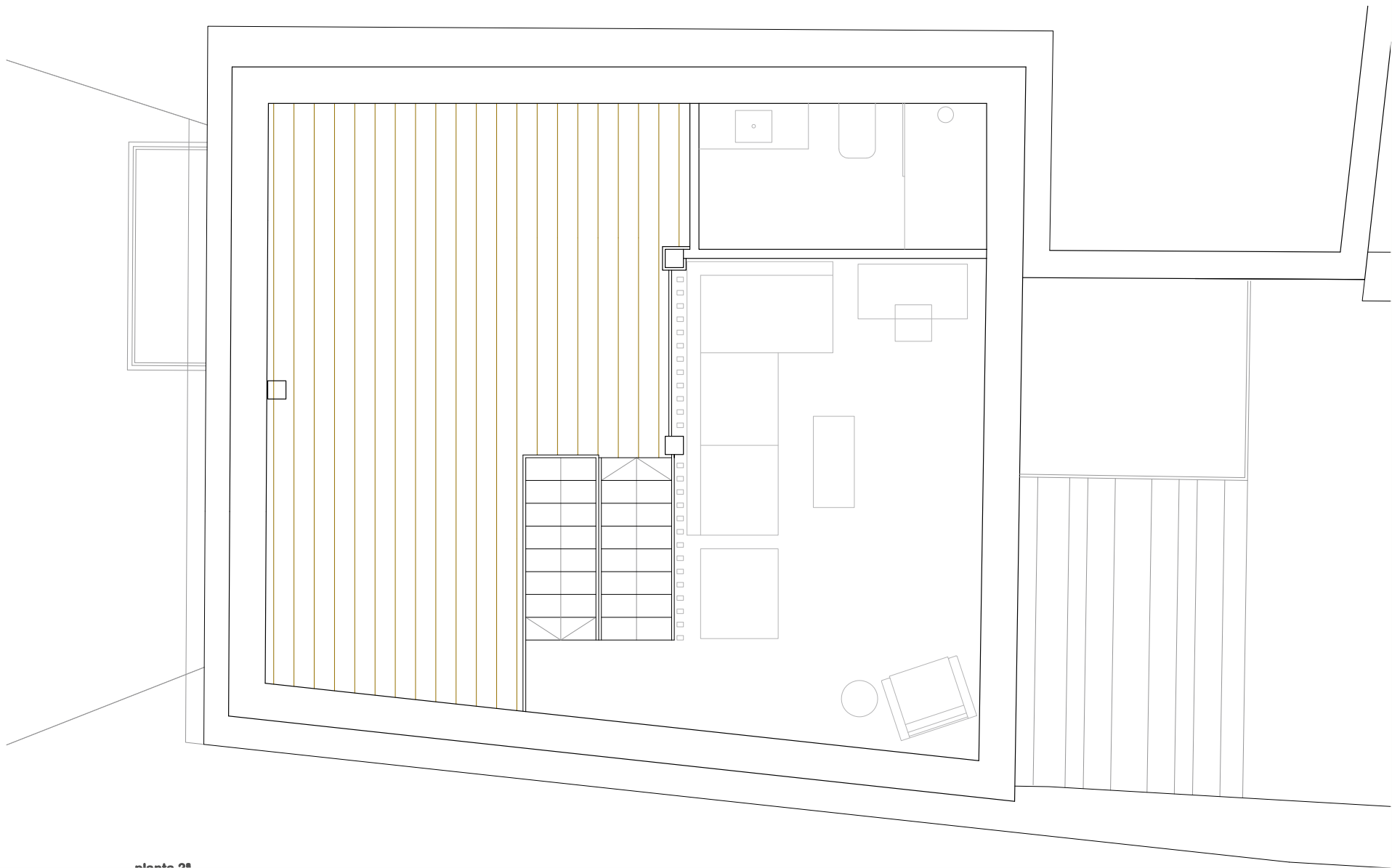
planta 2ª
